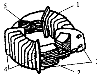
Рис. 63. Магнитная головка:
