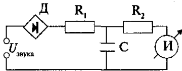
Рис. 46. Интегрирующая цепь измерителя уровня:
