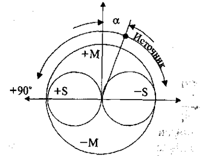
Рис. 32. Стереофоническая передача по системе MS
