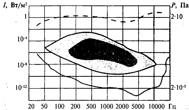
Рис. 3. Области слышимости: сплошная линия — порог слышимости; штриховая — болевой порог; светло-серым цветом обозначена область музыкальных звуков; темно-серым — речевых
