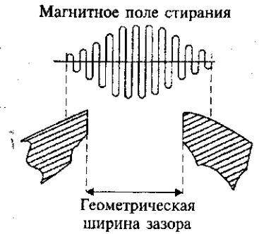
Рис. 69. Магнитное поле у зазора стирающей головки
