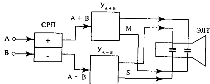
Рис. 51. Принципиальная схема стереогониометра
