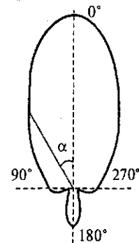
Рис. 20. Гиперкардиоид — характеристика остронаправленного микрофона
