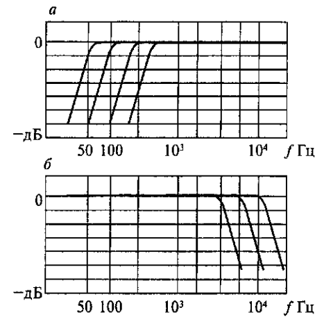
Рис. 43. Частотные характеристики фильтров:
