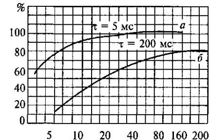
Рис. 47. Временные характеристики измерителя уровня
