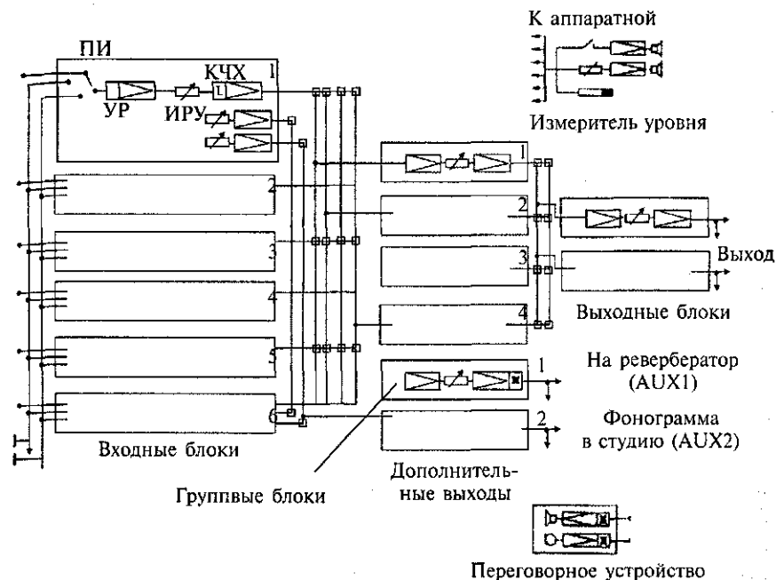
Рис. 38. Типовая блок-схема студийного микшерного пульта:
