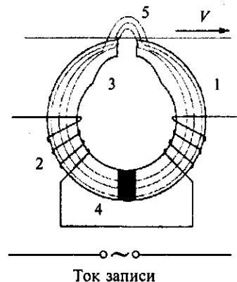
Рис. 64. Магнитная головка:
