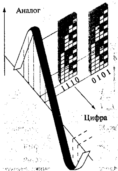
Рис. 86. Процесс квантования по уровню и цифрового кодирования
