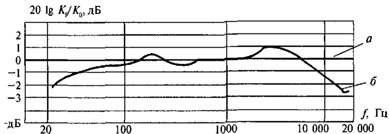
Рис. 10. Амплитудно-частотные характеристики:
