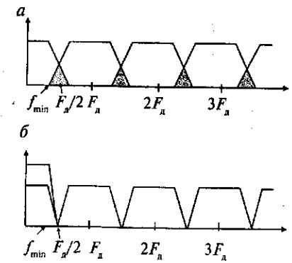
Рис. 85. Спектр дискретизованного сигнала:
