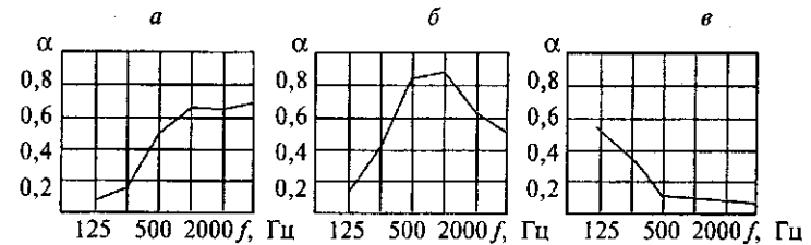
Рис. 1. Зависимость коэффициентов звукопоглощения от частоты: а — для пористых звукопоглощающих акустических плит; б — для перфорированных звукопоглотителей с наполнителем; в — для низкочастотных резонансных панелей
