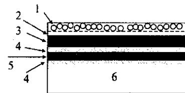
Рис. 92. Сечение мини-диска:
