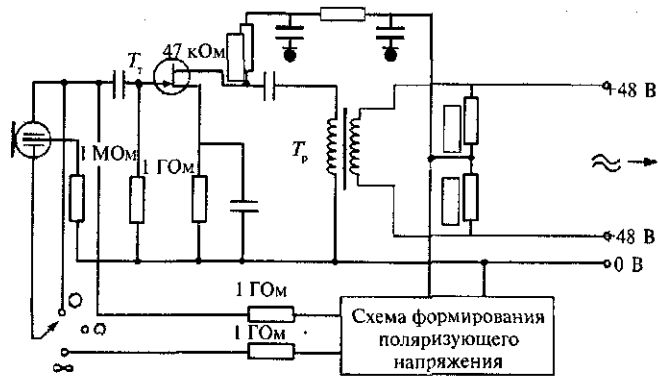
Рис. 29. Упрощенная схема переключения диаграмм направленности конденсаторного микрофона
