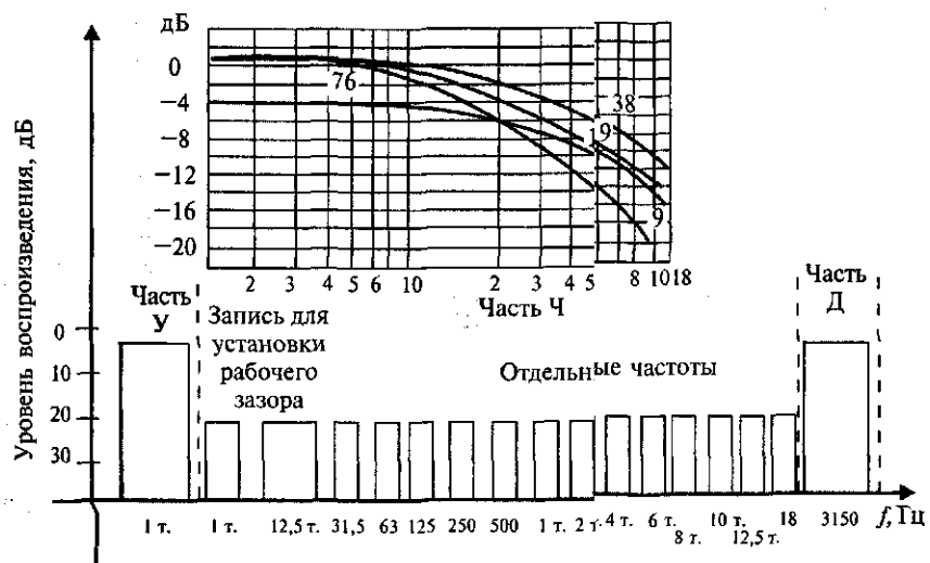
Рис. 82. Частотная характеристика ЛИМ
