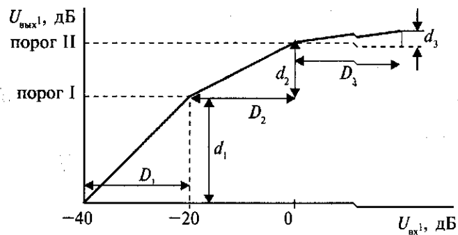
Рис. 42. Амплитудная характеристика компрессора-ограничителя, изображенная в логарифмическом масштабе
