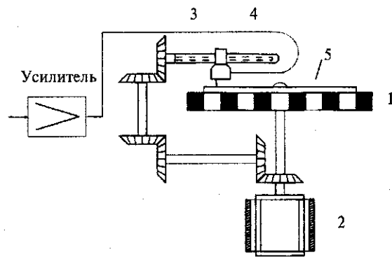
Рис. 56. Станок механической записи звука:
