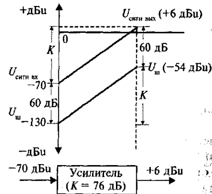
Рис. 14. Приведение шумов к входу усилителя на примере диаграммы уровней сигнала и шума для входа микрофонного усилителя
