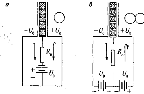
Рис. 28. Схема включения двухмембранного капсюля:
