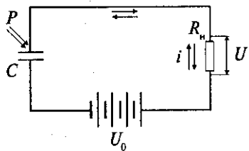
Рис. 25. Схема конденсаторного микрофона:
