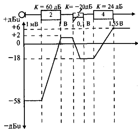
Рис. 9. Типичная диаграмма уровней: K — коэффициент усиления
