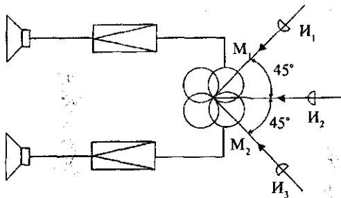
Рис. 31. Стерефоническая система XY
