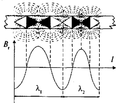
Рис. 65. Магнитная фонограмма при двух различных длинах волны
