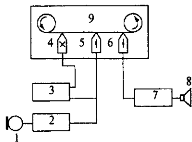
Рис. 62. Аппарат магнитной записи:
