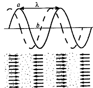
Рис. 2. Продольные звуковые волны
