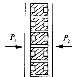
Рис. 26. Акустически комбинированный капсюль конденсаторного микрофона:
