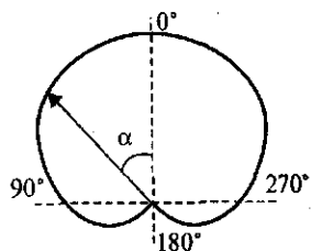
Рис. 19. Кардиоид — типичная диаграмма направленности односторонне направленного микрофона
