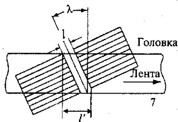
Рис. 80. Перекос рабочего зазора магнитной головки
