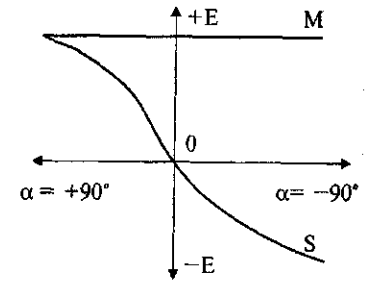
Рис. 33. Характеристики направленности микрофонной пары MS в прямоугольной системе координат
