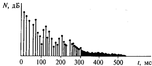
Рис. 7. Временная структура реверберационного процесса в помещении
