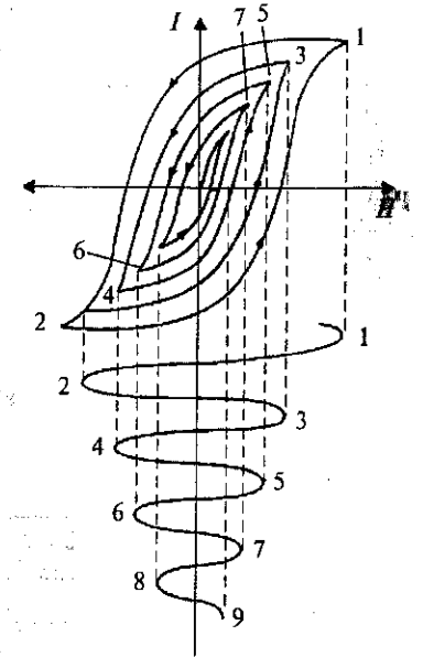
Рис. 70. Размагничивание полем высокой частоты
