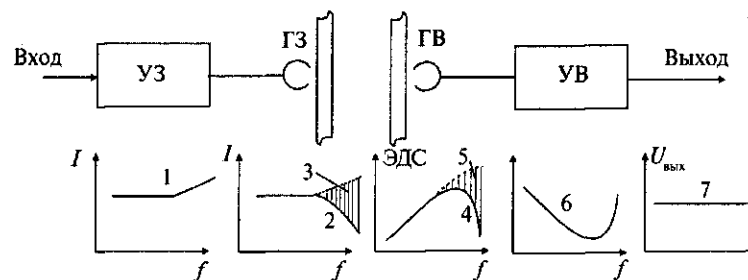
Рис. 79. Частотная коррекция в сквозном канале:
