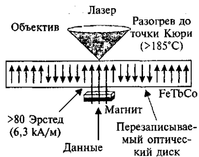
Рис. 93. Запись на мини-диск
