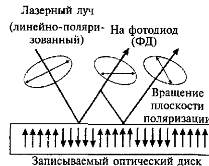
Рис. 94. Считывание записываемого диска MD-R
