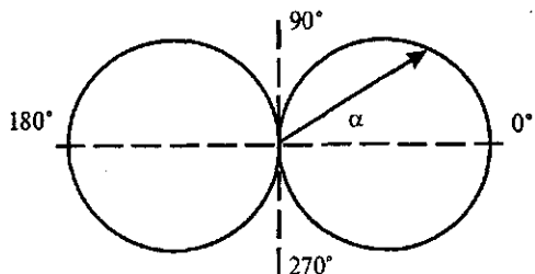
Рис. 18. Диаграмма направленности двустороннего микрофона
