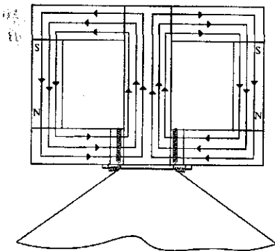
Рис. 54. Магнитная и подвижная системы динамика. (Стрелками указаны силовые линии постоянного магнитного поля.)
