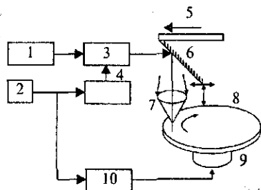
Рис. 90. Оптическая запись на компакт-диск:
