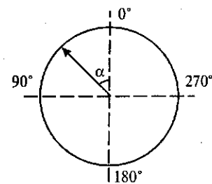
Рис. 16. Идеализированная диаграмма направленности микрофона ненаправленного действия
