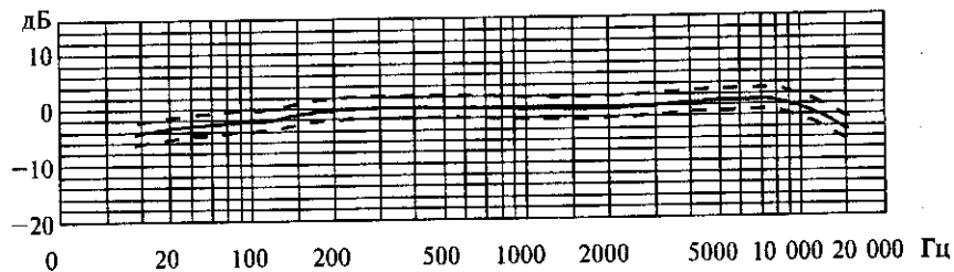
Рис. 15. Частотная характеристика микрофона
