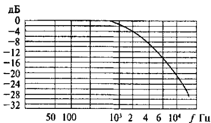
Рис. 75. Частотная характеристика магнитной записи
