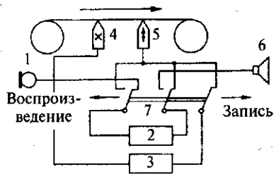
Рис. 67. Бытовой магнитофон с универсальным усилителем:
