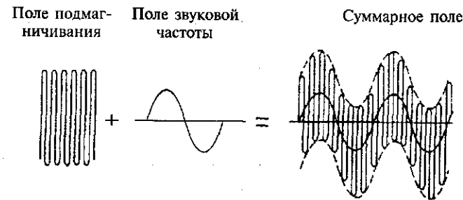
Рис. 73. Суммирование полей подмагничивания звука. (Соотношение размахов полей условно. Поле подмагничивания превышает звуковое в 10 раз.)
