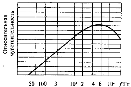
Рис. 78. Частотная характеристика канала записи—воспроизведения без коррекции
