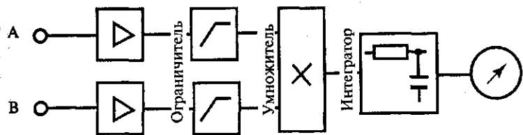
Рис. 50. Принципиальная схема коррелометра
