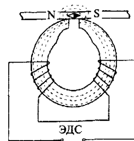
Рис. 66. Воспроизведение фонограммы с магнитной ленты
