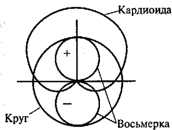
Рис. 23. Формирование кардиоиды
