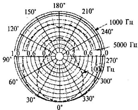
Рис. 17. Зависимость диаграммы направленности от частоты звукового сигнала
