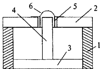
Рис. 24. Динамический (катушечный) микрофон:
