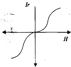
Рис. 72. Остаточная намагниченность как функция магнитного поля
