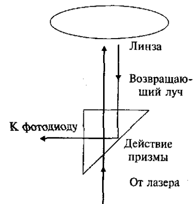
Рис. 91. Упрощенная схема считывания информации с компакт-диска
