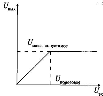
Рис. 39. Идеализированная амплитудная характеристика усилителя-ограничителя в линейном масштабе
