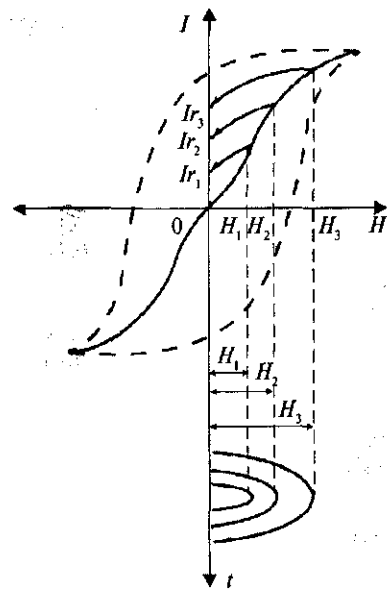
Рис. 71. Намагничивание ленты
