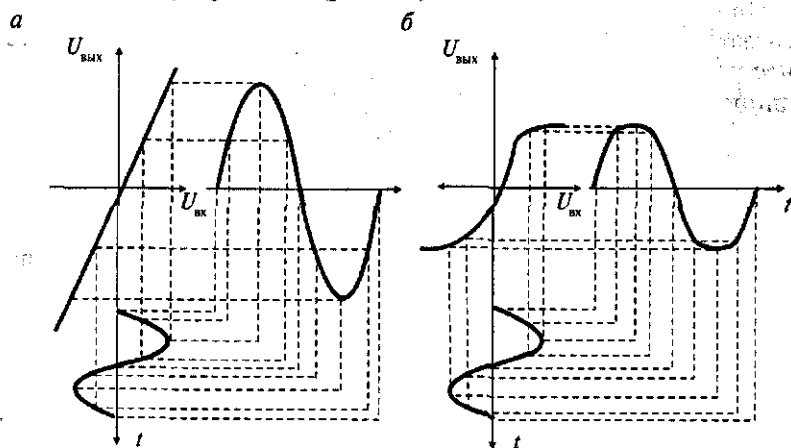
Рис. 11. Нелинейные искажения:
