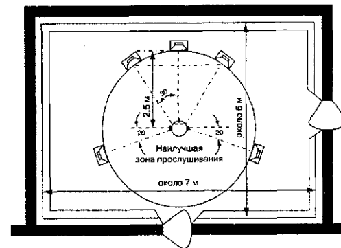
Рис. 37. Стандартное расположение громкоговорителей по системе 5.1 (без сабвуфера)
