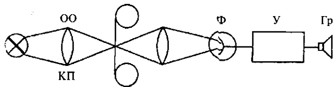
Рис. 58. Воспроизведение фонограммы кинофильма: лампа ОО — оптическая система; КП — киноплёнка; Ф — фотоприемник; У — усилитель; Гр — громкоговоритель
