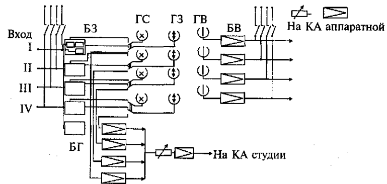
Рис. 83. Блок-схема многодорожечного магнитофона
