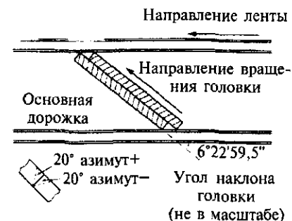
Рис. 89. Формат DAT
