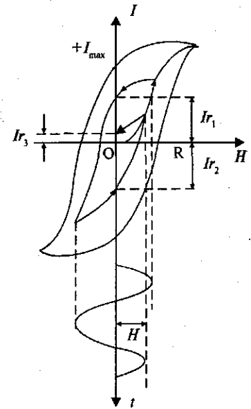
Рис. 61. Частные циклы перемагничивания
