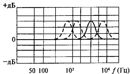
Рис. 45. Частотная характеристика фильтра присутствия
