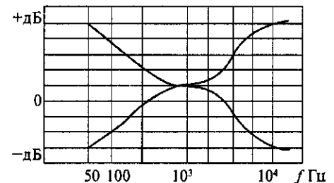
Рис. 44. Частотные характеристики параметрического эквалайзера
