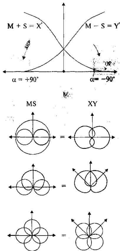
Рис. 34. Преобразование информации системы MS в информацию системы XY: график зависимости выходных напряжений от углов падения волны после суммарно-разностного преобразования; переход от системы MS к системе XY
