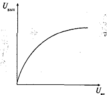
Рис. 40. Амплитудная характеристика компрессора в линейном масштабе
