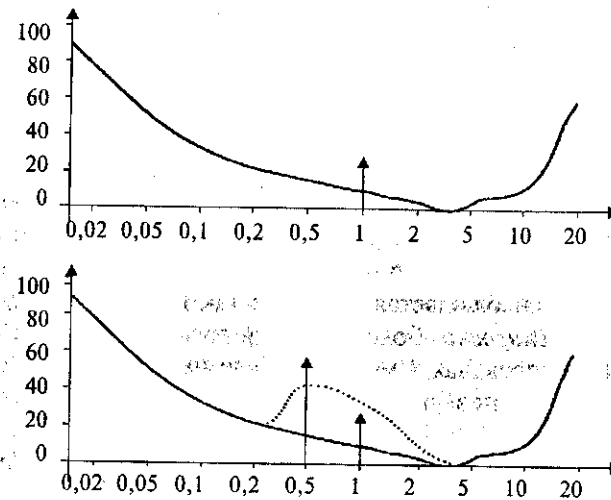
Рис. 95. Психоакустический эффект маскировки сигналов
