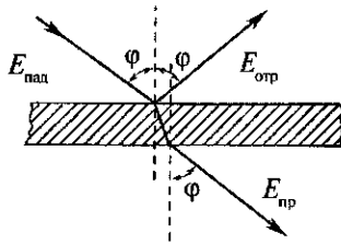
Рис. 6. Преломление и отражение звуковой волны
