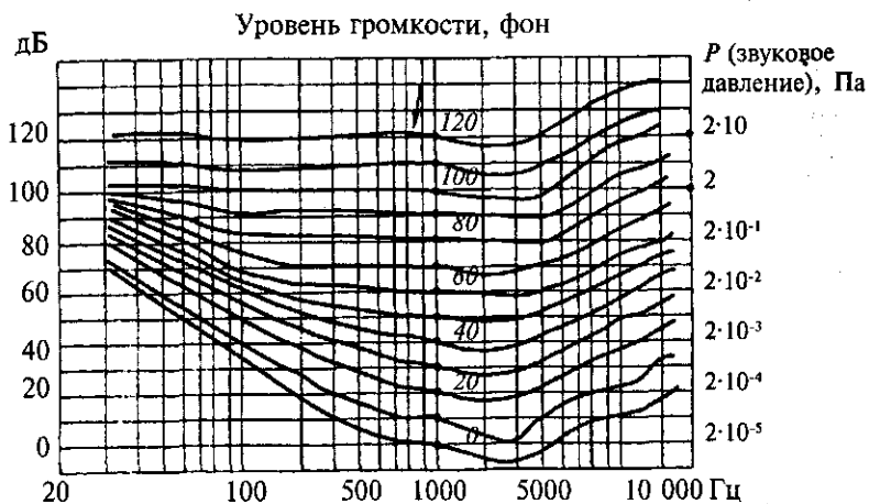
Рис. 4. Кривые равной громкости
