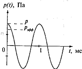
Рис. 1. Звуковое давление как функции времени. Зависимость от координат точки наблюдения скрыта в начальной фазе колебания
