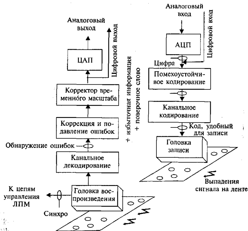
Рис. 87. Структурная схема цифрового магнитофона
