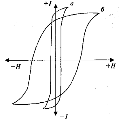
Рис. 60. Петля гистерезиса (условно): a — магнитомягкого материала; б — магнитожесткого материала
