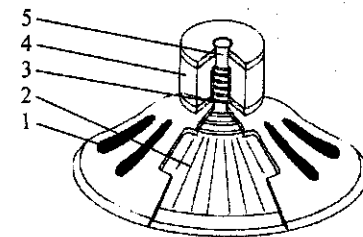
Рис. 53. Конструкция электродинамического громкоговорителя: 1 — диффузордержатель; 2 — диффузор; 3 — звуковая катушка; 4 — постоянный магнит; 5 — цилиндрический керн
